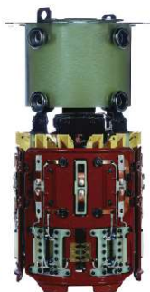
◀ ZM有载分接开关 芯子
